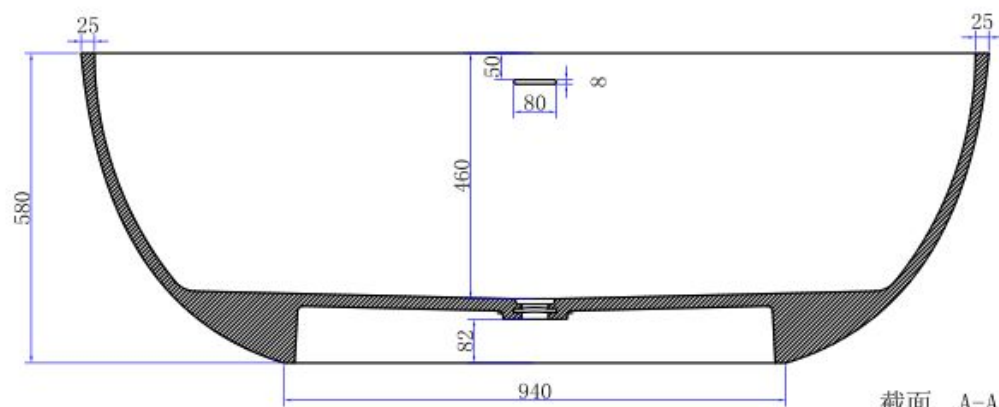
截面 A-A
