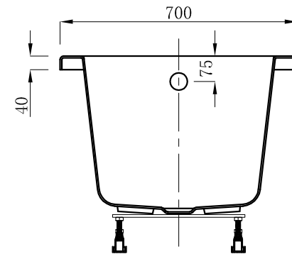
截面 G-G
