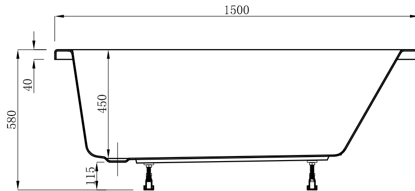
截面 F-F
