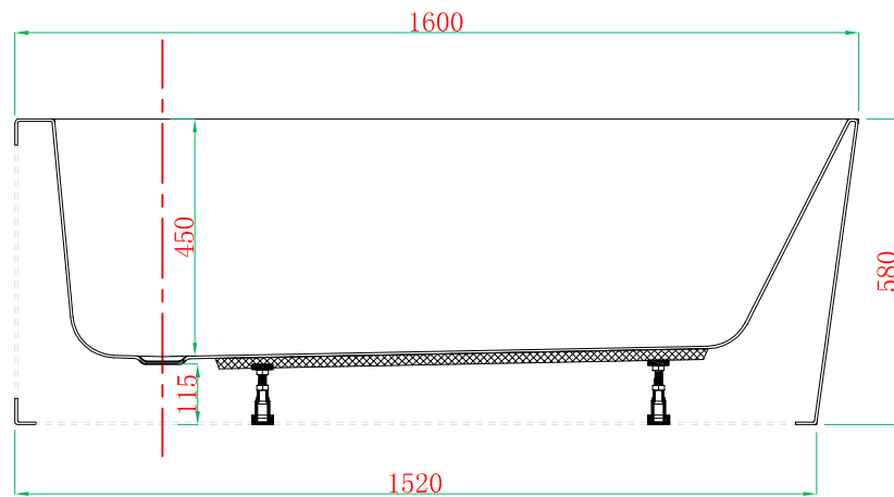
截面 Section AA
