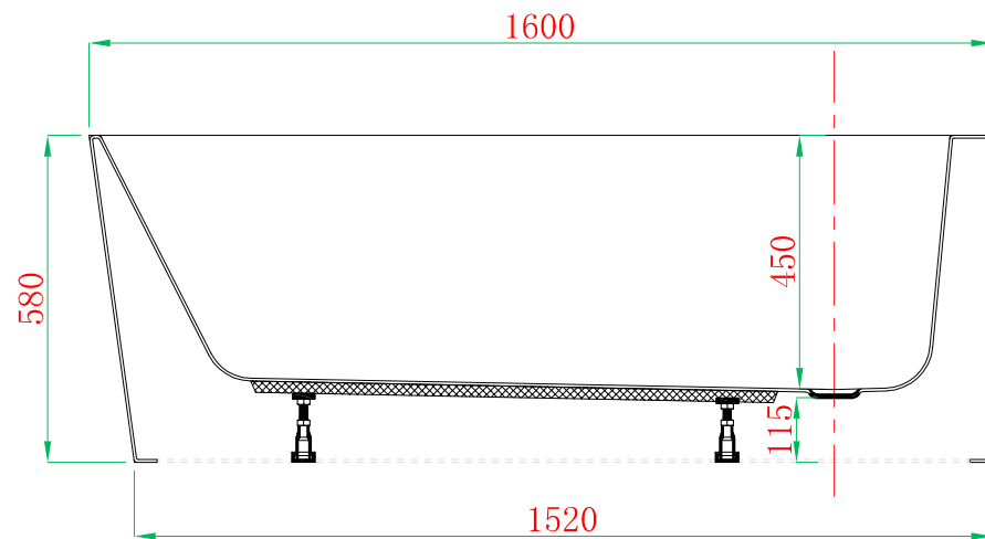
截面 Section AA
