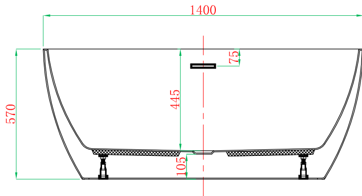
F-F 剖视图
