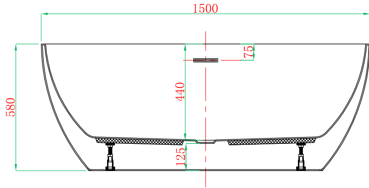
F-F 剖视图
