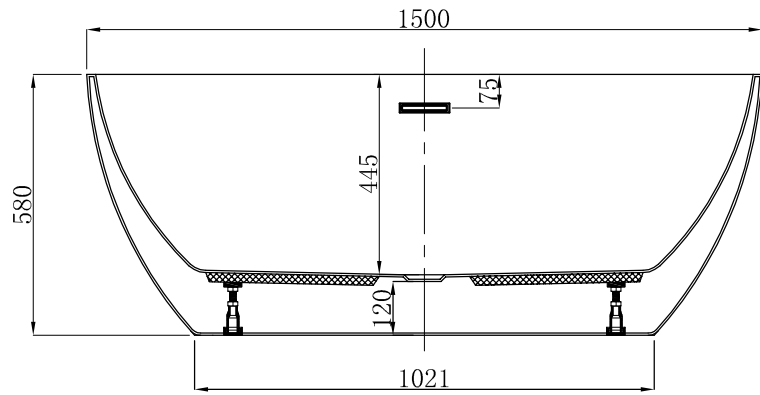
F-F 剖视图
